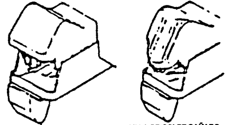
CONDICIÓN NORMAL DE LA VARILLA DE GOLPE, ES DECIR, NO HAY EVIDENCIA DE DAÑO COMO RESULTADO DEL CONTACTO CON EL BRAZO DE CONTROL SUPERIOR.
